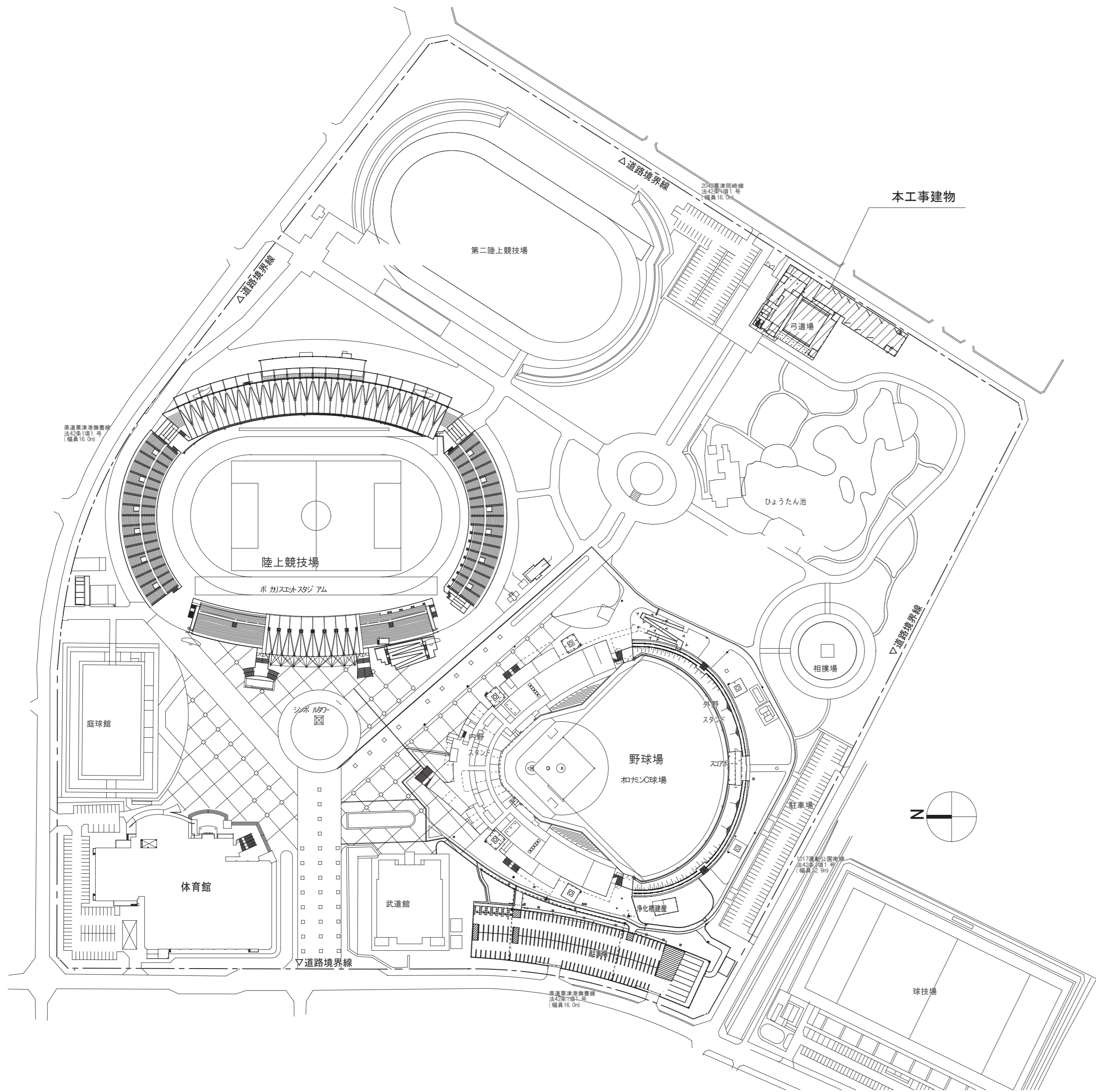
配置図 S=1/2000
